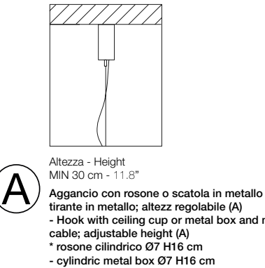
A Altezza - Height MIN 30 cm - 11.8" Aggancio con rosone o scatola in metallo e tirante in metallo; altezza regolabile (A) - Hook with ceiling cup or metal box and metal cable; adjustable height (A) * rosone cilindrico Ø7 H16 cm - cylindric metal box Ø7 H16 cm
