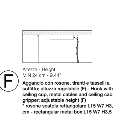
F Altezza - Height MIN 24 cm - 9.44" Aggancio con rosone, tiranti e tasselli a soffitto; altezza regolabile (F) - Hook with ceiling cup, metal cables and ceiling cable gripper; adjustable height (F) * rosone scatola rettangolare L15 W7 H3,5 cm - rectangular metal box L15 W7 H3,5 cm
