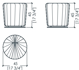
BD 71 ottoman - pouf - ottomane - pouf - Круглый пуф
